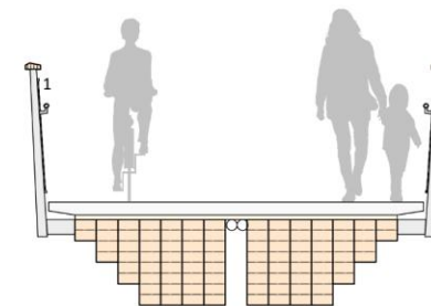
Skizze Querschnitt M 1:50
