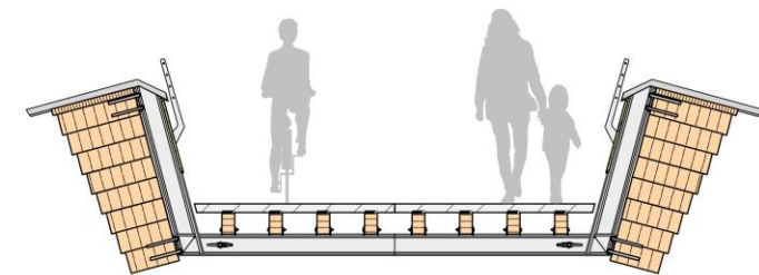
Skizze Querschnitt M 1:50
