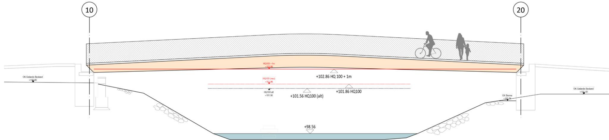
Skizze Längsschnitt M 1:100
