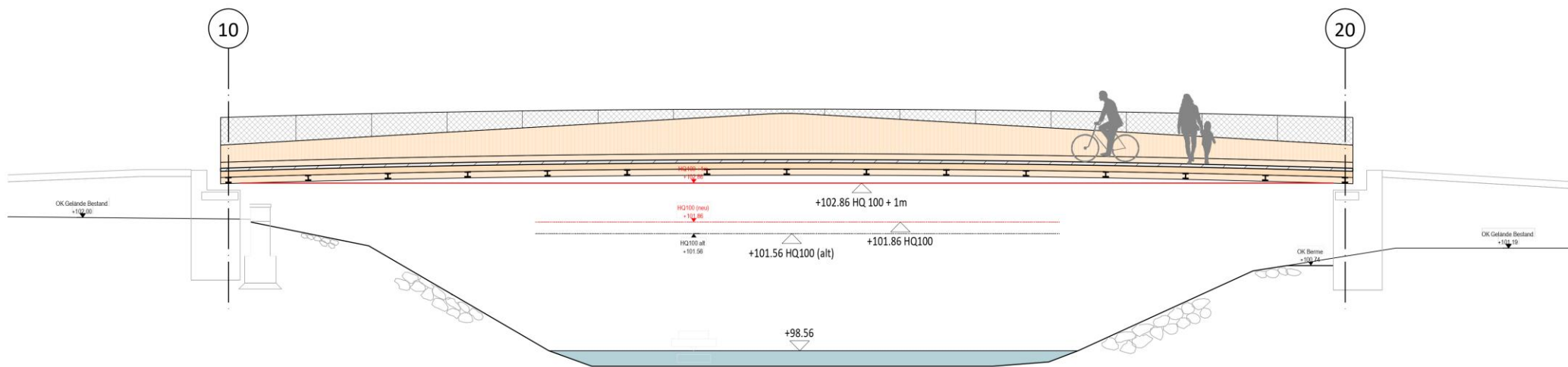
Skizze Längsschnitt M 1:100
